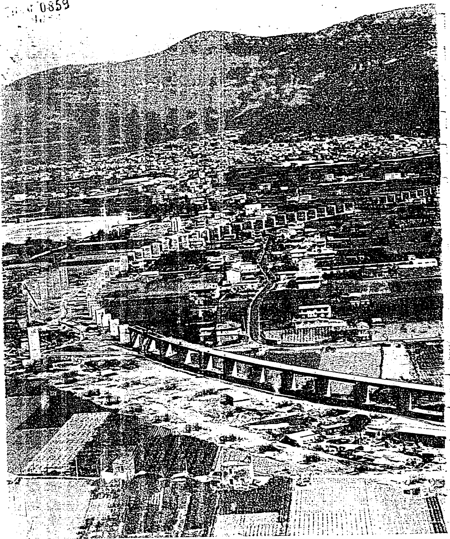
Primo tratto della linea ferroviaria a doppio binario a Monte del Vesuvio First section of the Monte del Vesuvio double-track line Premier tronçon de la ligne à voie double à Monte del Vesuvio
