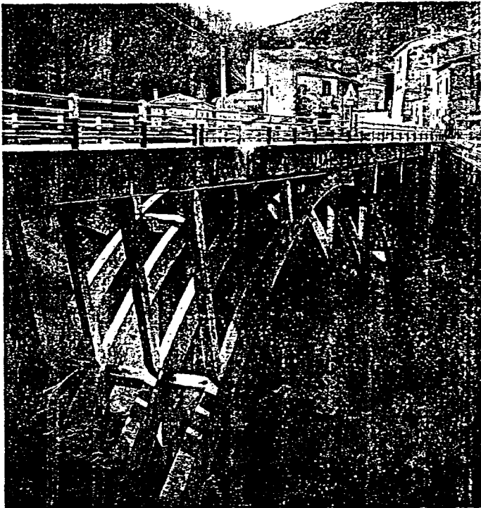
Strada e ponte in Valnerina, 1953-55 Road and bridge in Valnerina, 1953-55 Route et pont dans la Valnerina, 1953-55
