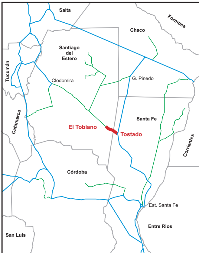
Esquema de ubicación del tramo Tostado - El Tobiano respecto de la red de Belgrano Cargas y Logística S.A. - Línea Belgrano (plano parcial de la red)
