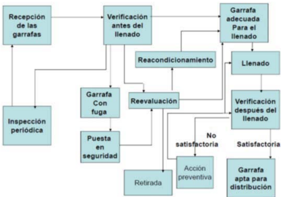
DIAGRAMA de FLUJO de las VERIFICACIONES ANTES, DURANTE y DESPUES de LLENADO
