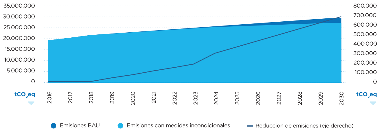
Figura 35. Evolución de las emisiones de gases de efecto invernadero y reducción de emisiones a partir del Programa Transporte Inteligente (sin capacitación) (2016-2030).
