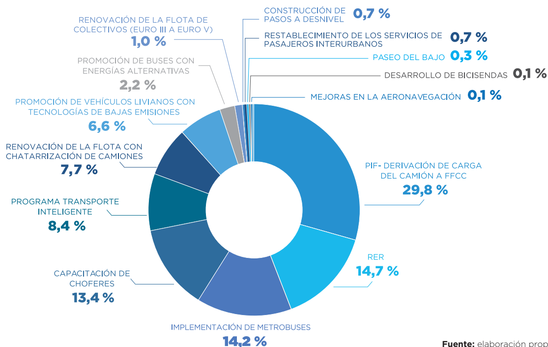
Figura 21. Ahorro de cada medida de mitigación según el aporte en 2030.
