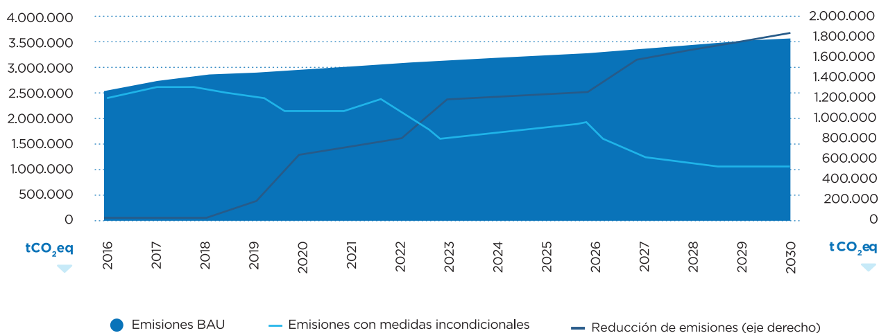
Figura 34. Evolución de las emisiones de gases de efecto invernadero y reducción de emisiones a partir del Plan de Inversión Ferroviaria de Cargas (2016-2030).
