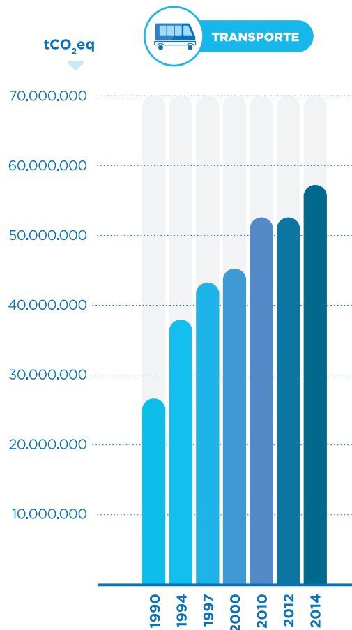
Figura 15. Evolución histórica de las emisiones del subsector transporte (1990-2014).
