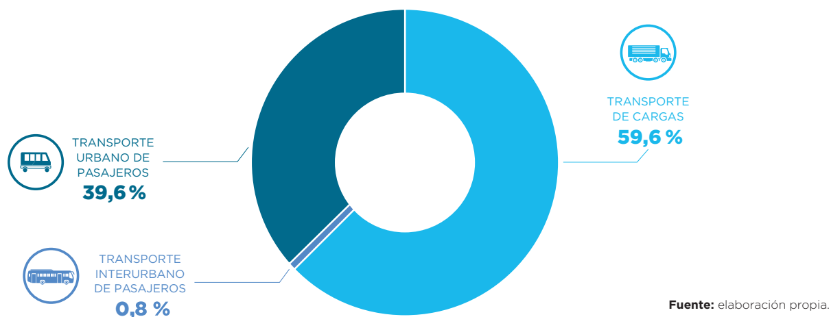
Figura 20. Participación de las acciones de mitigación en el ahorro acumulado del sector transporte (2011-2030).
