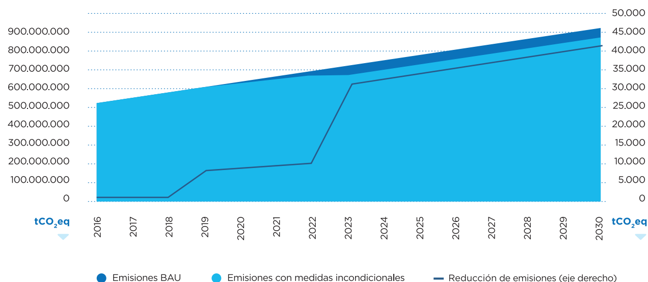
Figura 26. Evolución de las emisiones de gases de efecto invernadero y reducción de emisiones a partir de la construcción de pasos a desnivel (2016-2030).
