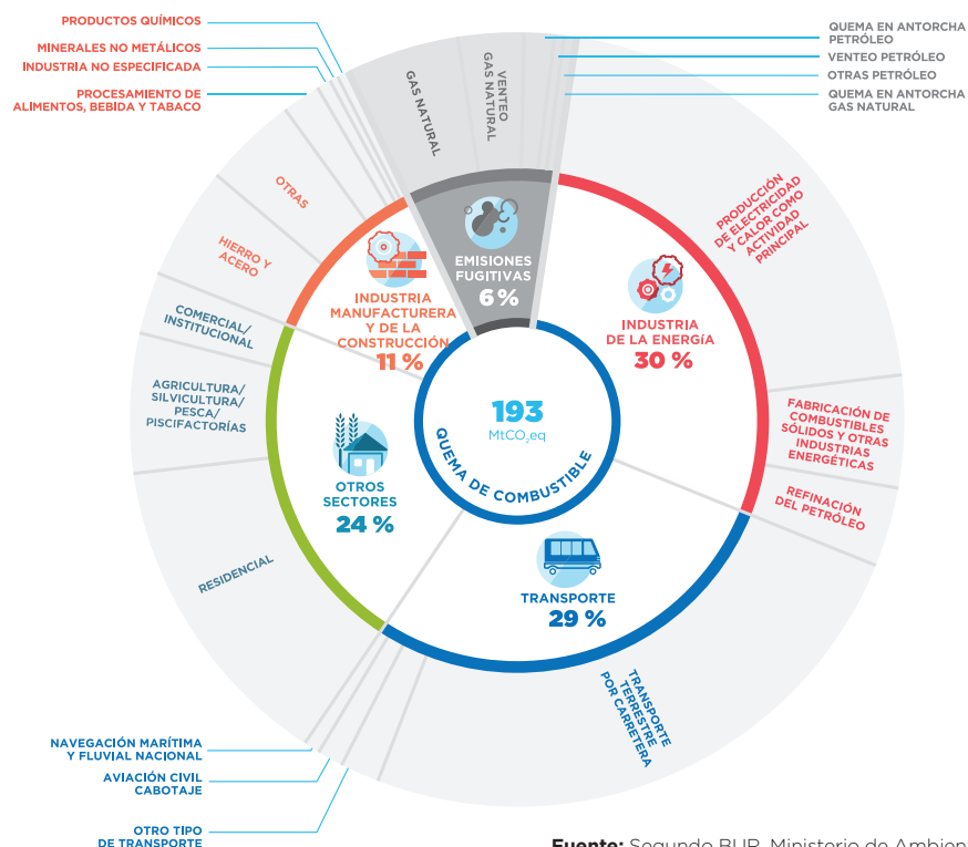
Figura 14. Inventario del sector energía (2014).
