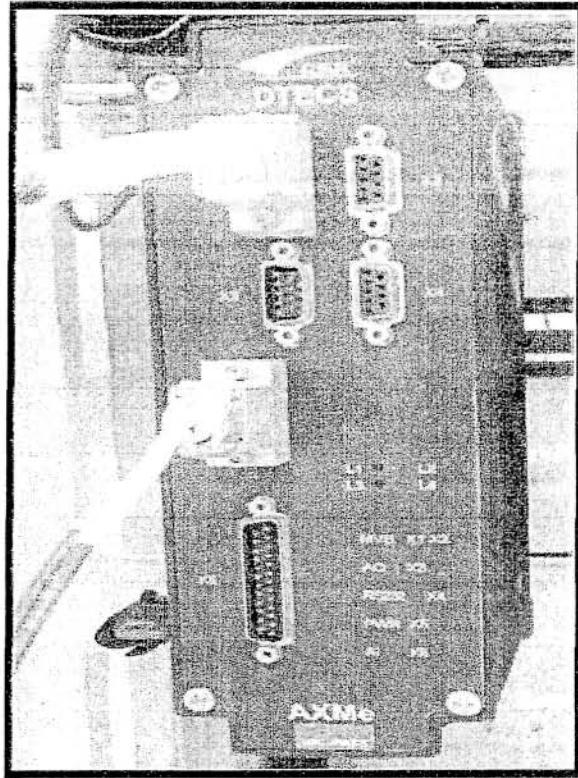
G122 Digital input module
