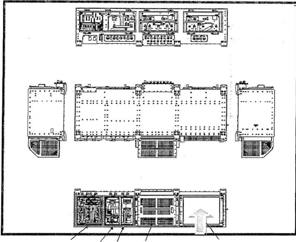
G98 Power module
