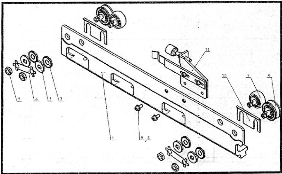
C44 Conjunto de carro de rodamiento (izquierdo)
