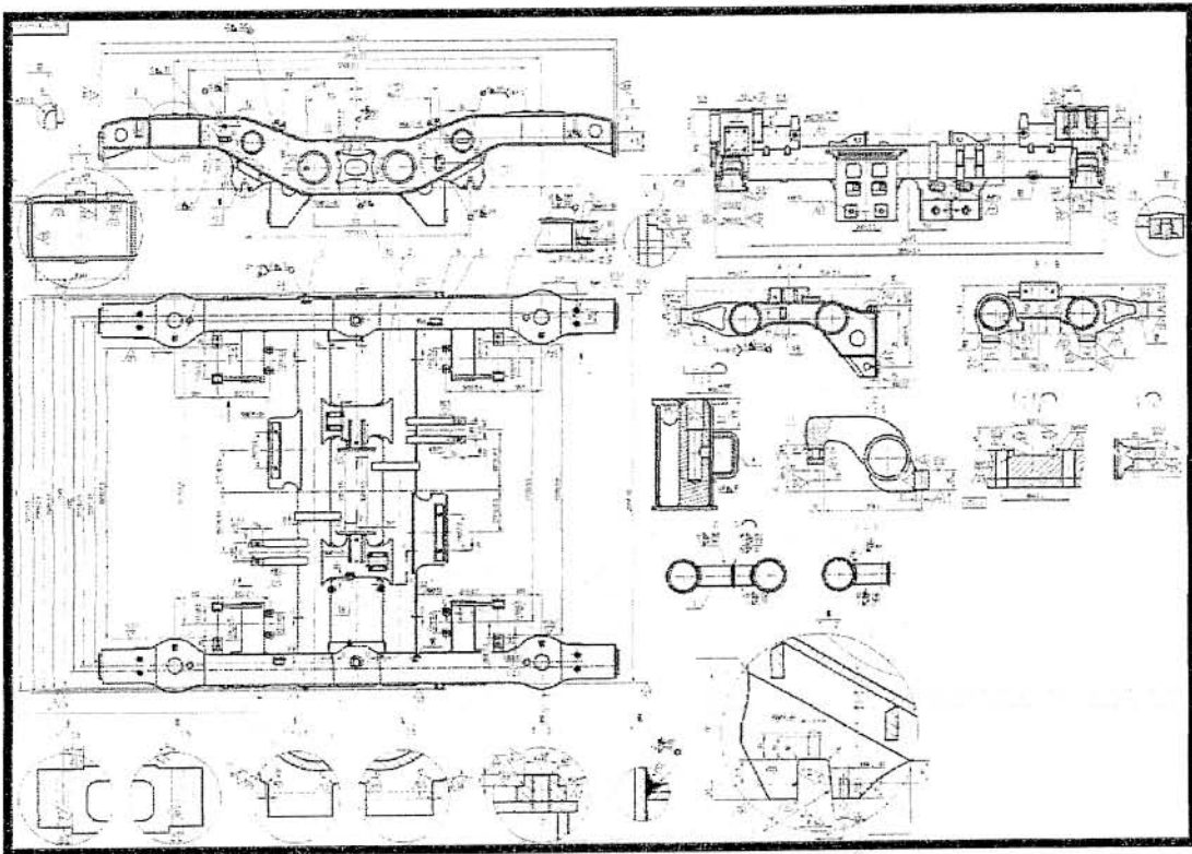
F65 Conjunto de bastidor de remolque
