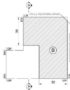
PLANTA TIPO 3°- 11° PISO 2437,70m2
